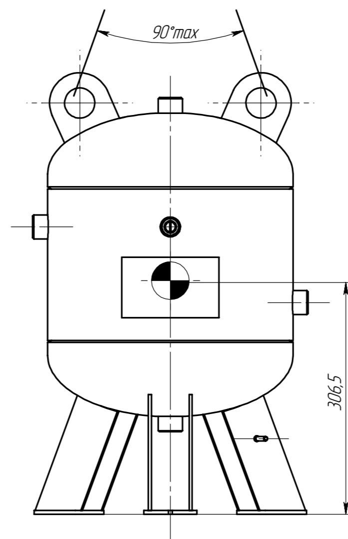
Схема строповки (1:5)
