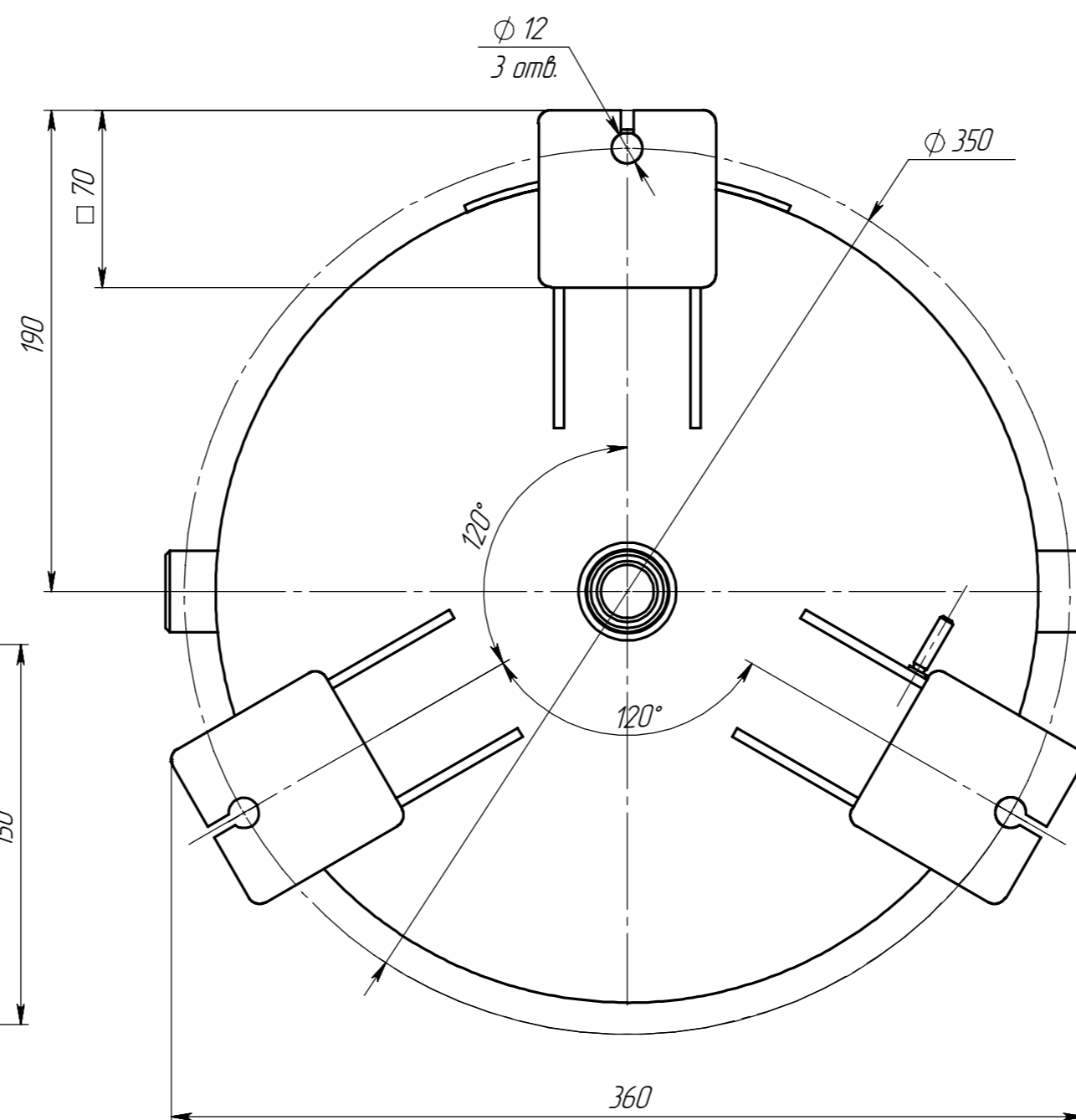
Схема строповки (1:5)
