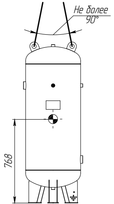
Схема строповки аппарата в вертикальном положении
